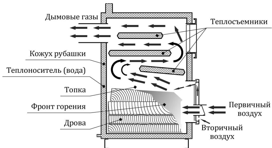
Рисунок 3 – Схема КОД-20ГТ, КОД-25ГТ, КОД-30ГТ, КОД-35ГТ, КОД-40ГТ
