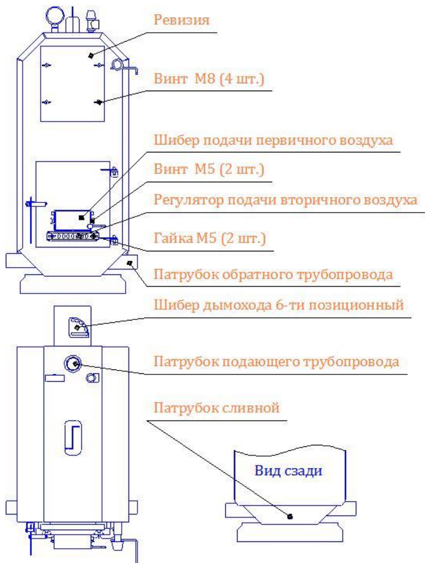
Рисунок 7 – Основные элементы котла с горизонтальной дымовой трубой
