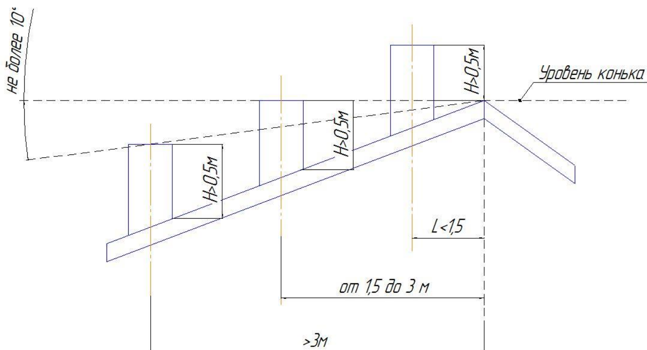
Рисунок 11 – Варианты расположения трубы на скате
