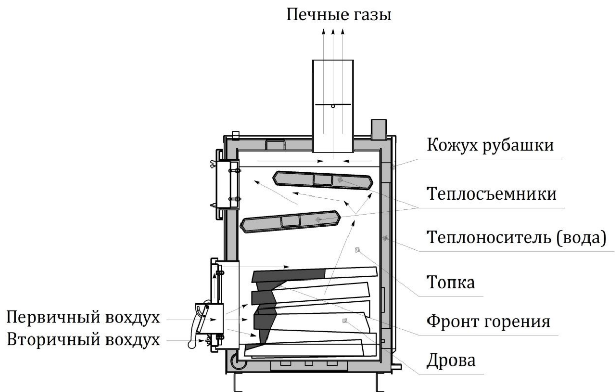
Рисунок 1 – Схема КОД-18
