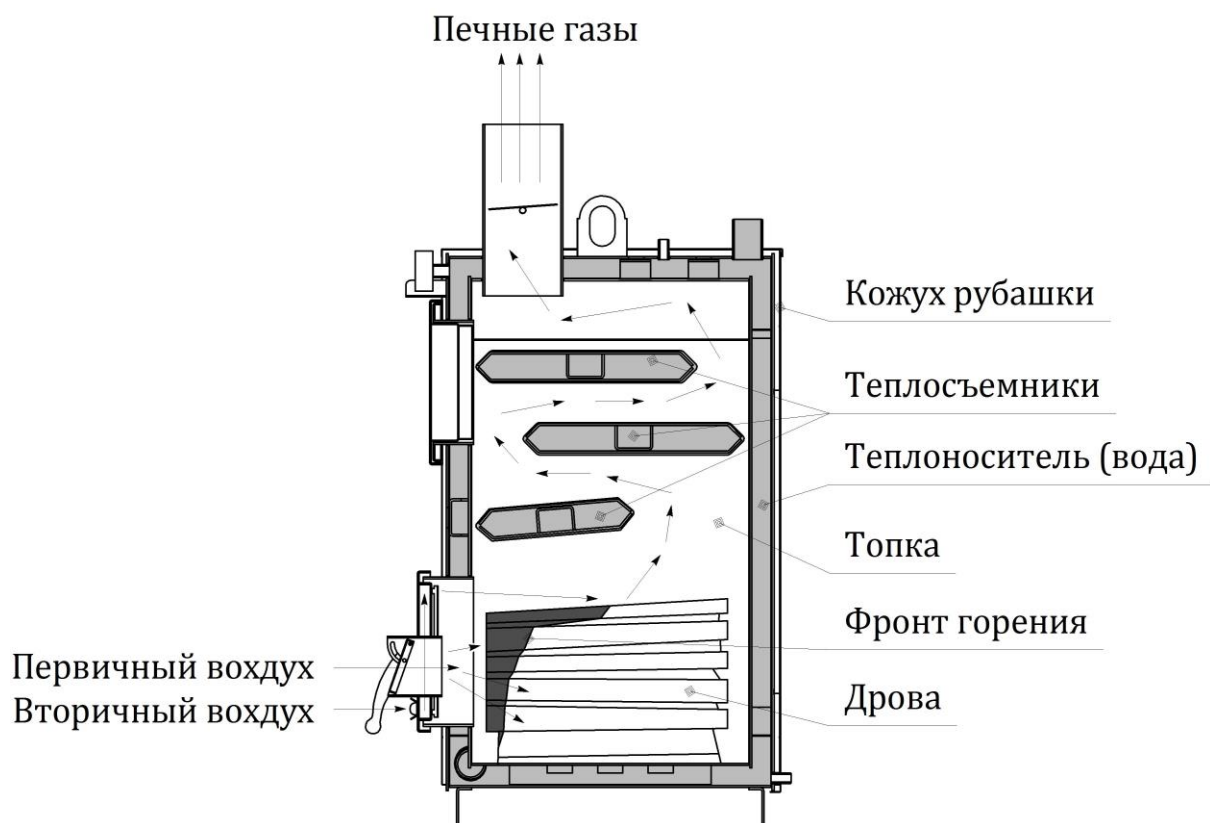
Рисунок 2 – Схема КОД-20, КОД-25, КОД-30, КОД-35, КОД-40
